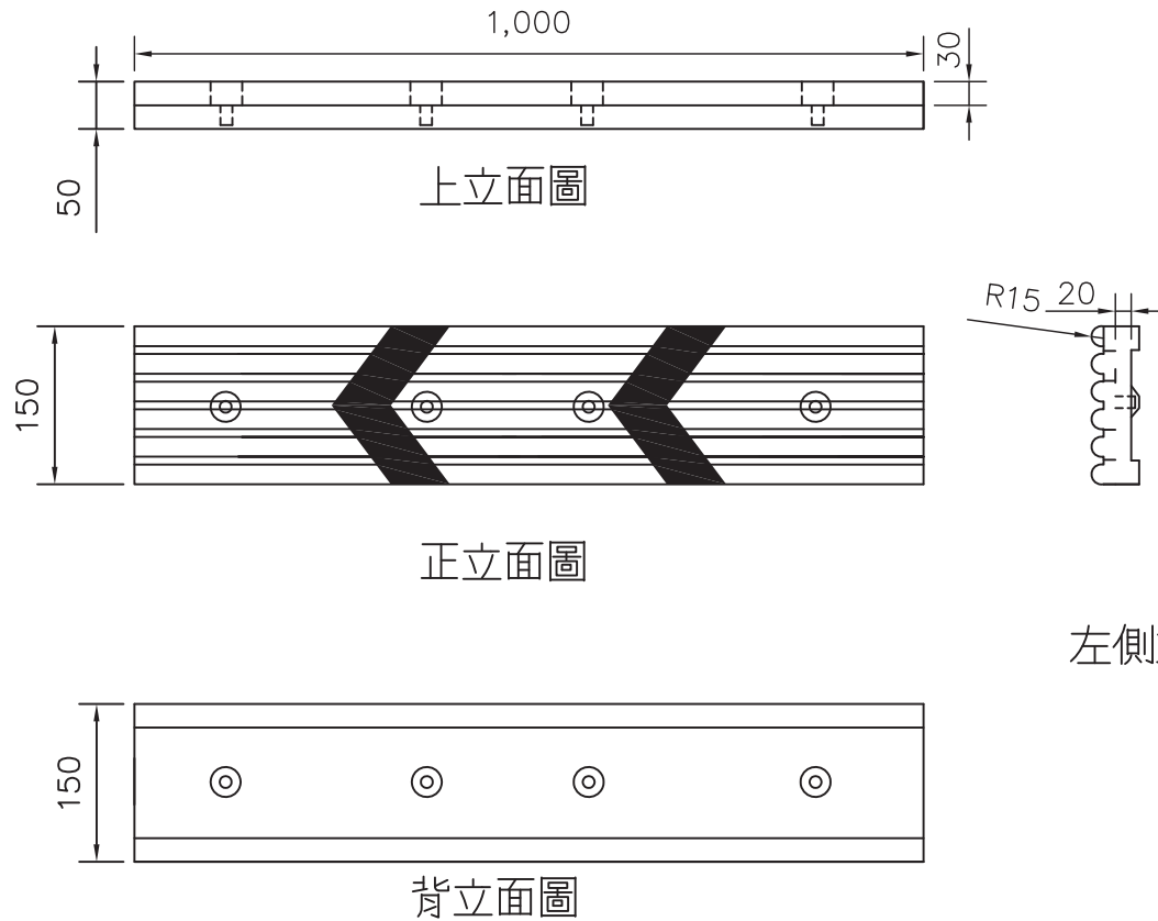
橡膠警示防護條尺寸圖 (寬 150 長 1000 厚 50)(單位M/M±5%)
